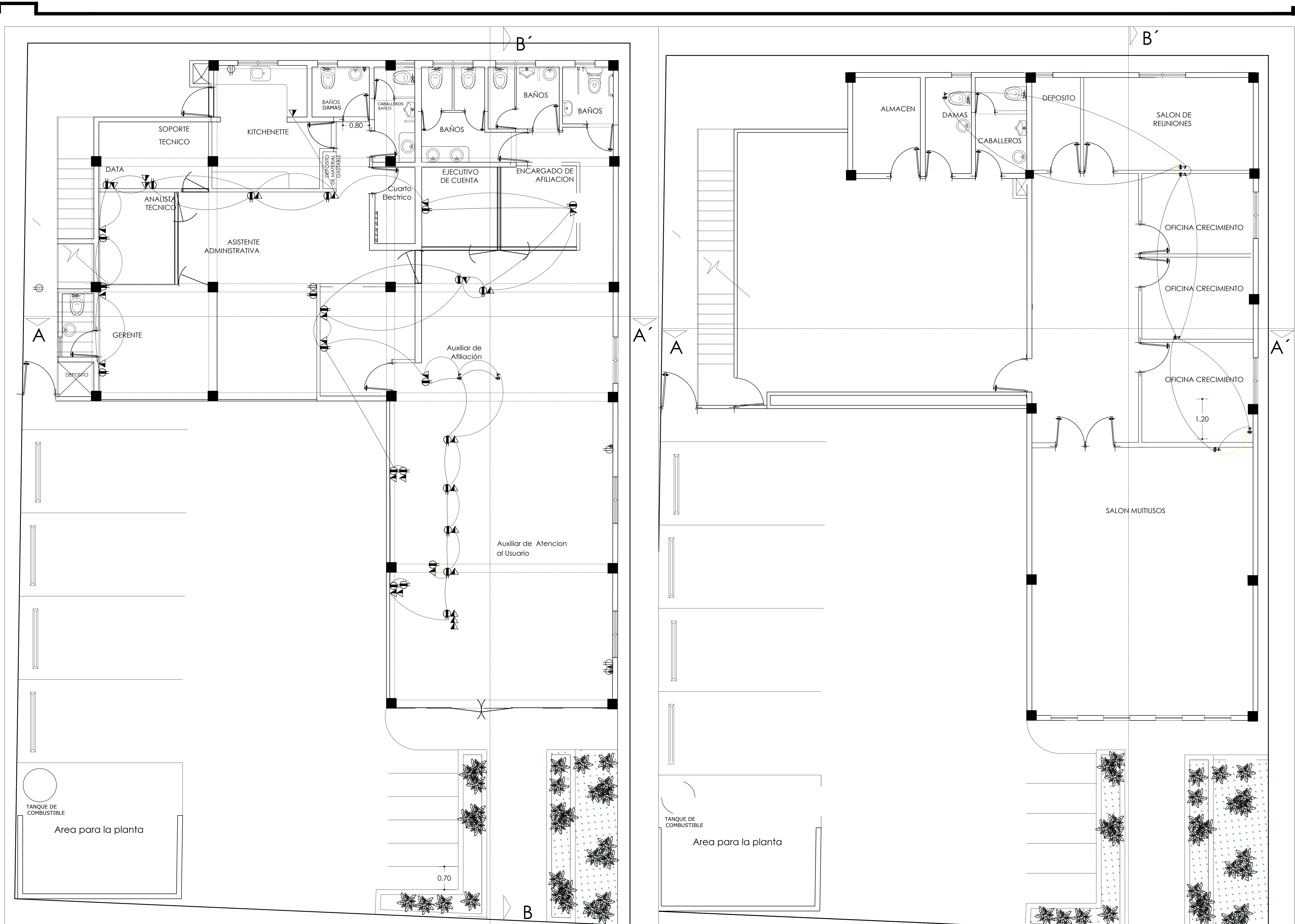
PLANTA DATA Y UPS 1ER Y 2DO NIVEL Escala: Indicada
