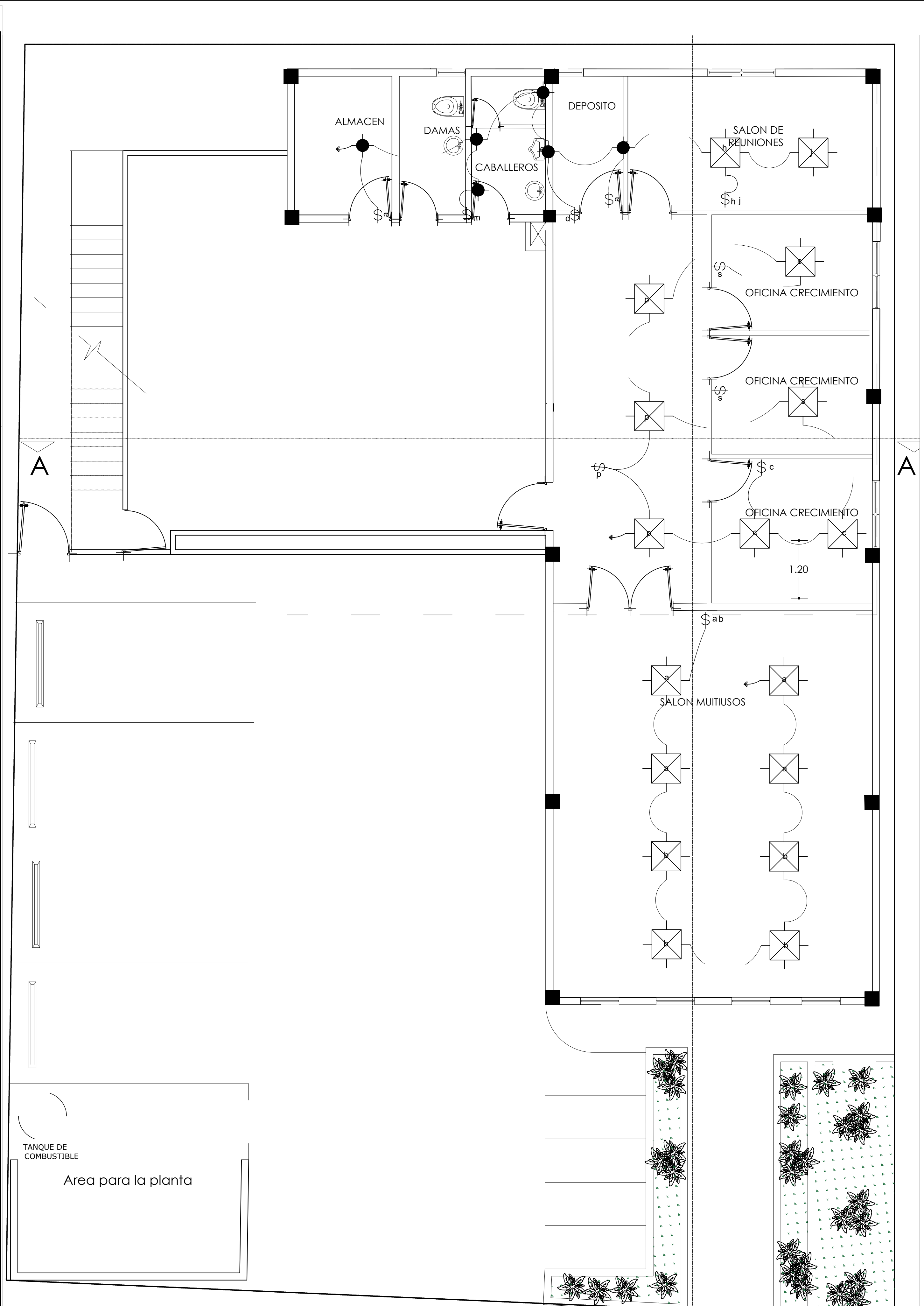
PLANTA ILUMINACION 2DO NIVEL Escala: Indicada
