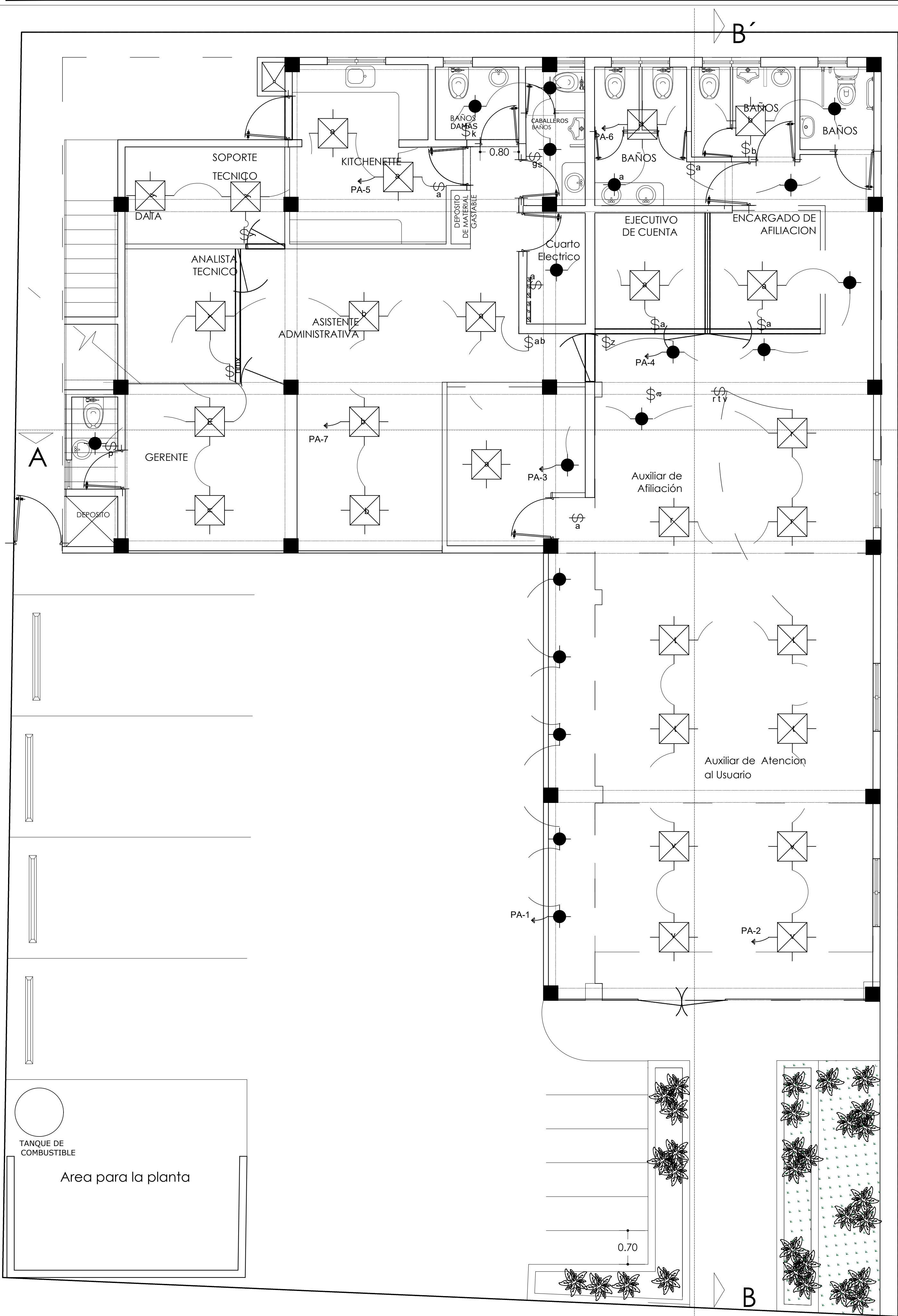
PLANTA ILUMINACION 1ER NIVEL Escala: Indicada
