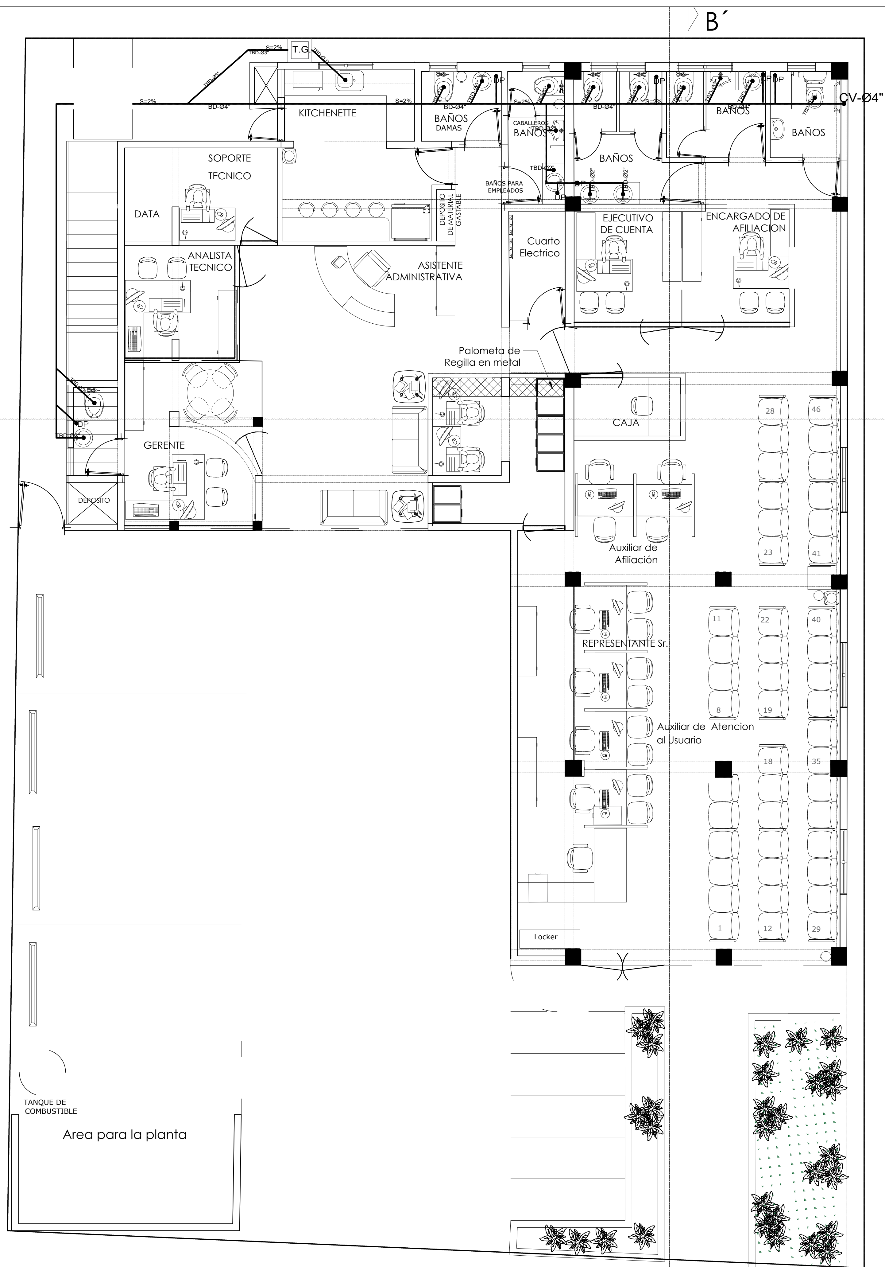
PLANTA SANITARIA PRIMER NIVEL
