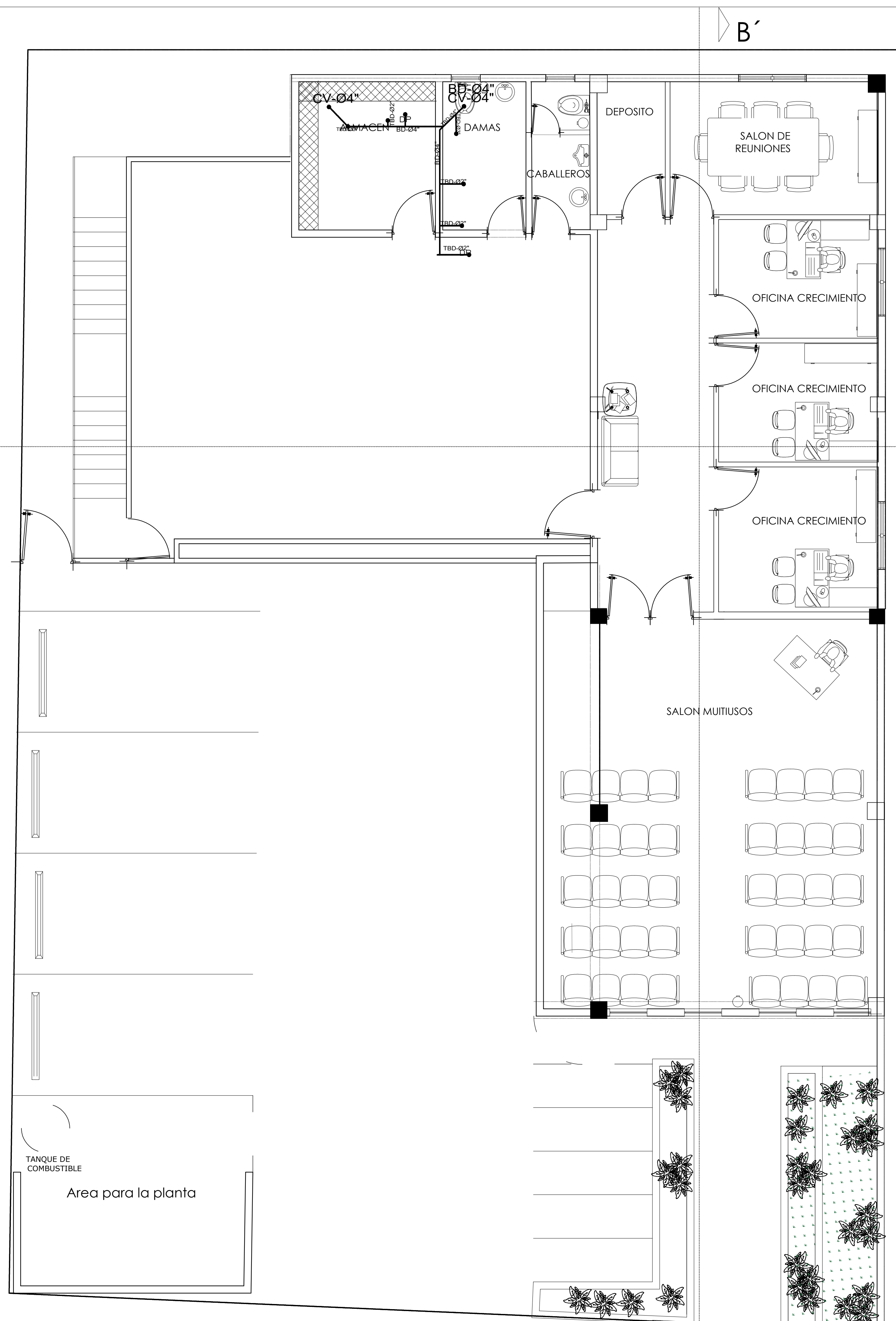
PLANTA SANITARIA SEGUNDO NIVEL
