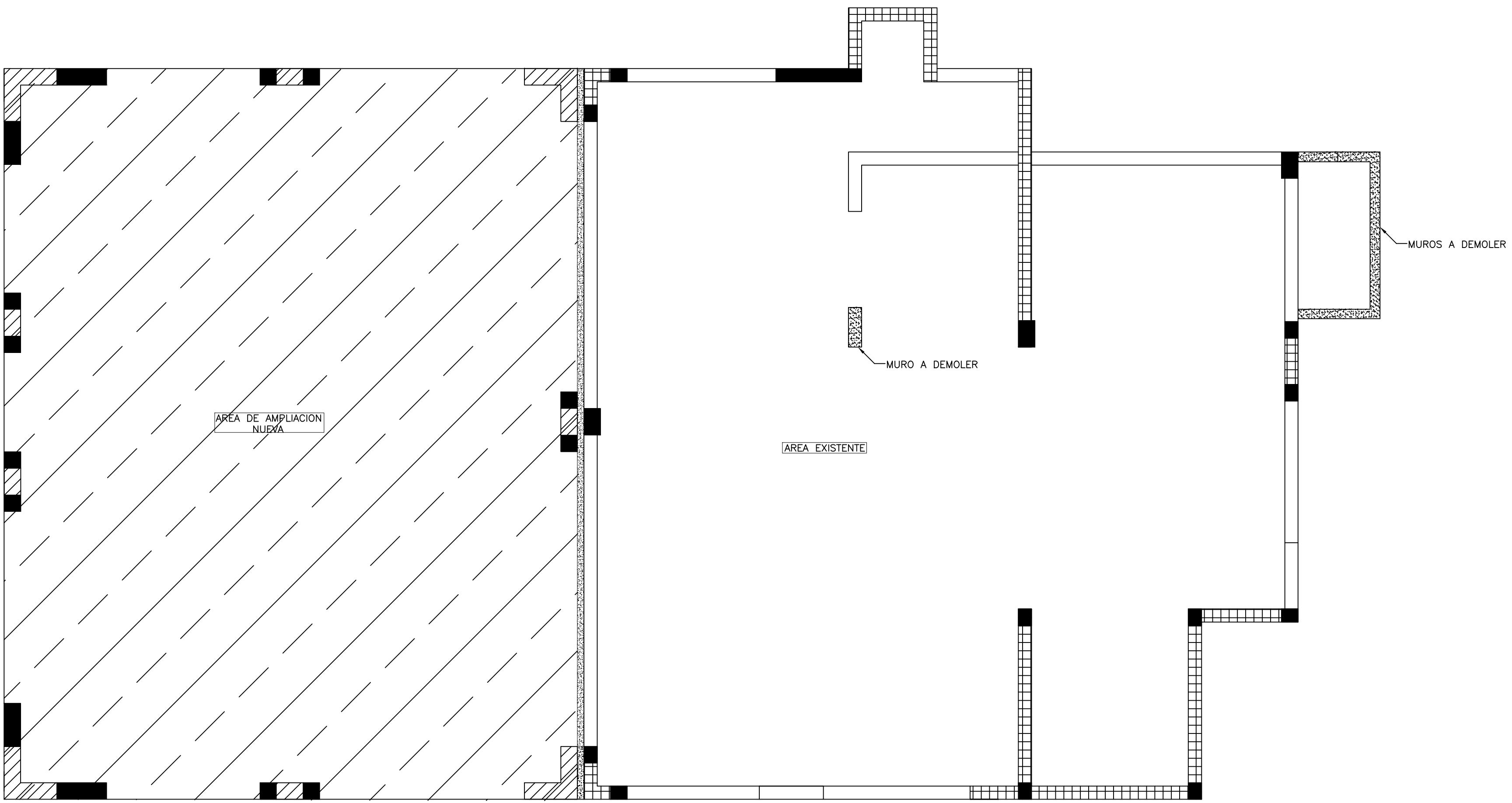
1 IDENTIFICACION DE ELEMENTOS A DEMOLER Y REFORZAR ESC. 1:50
