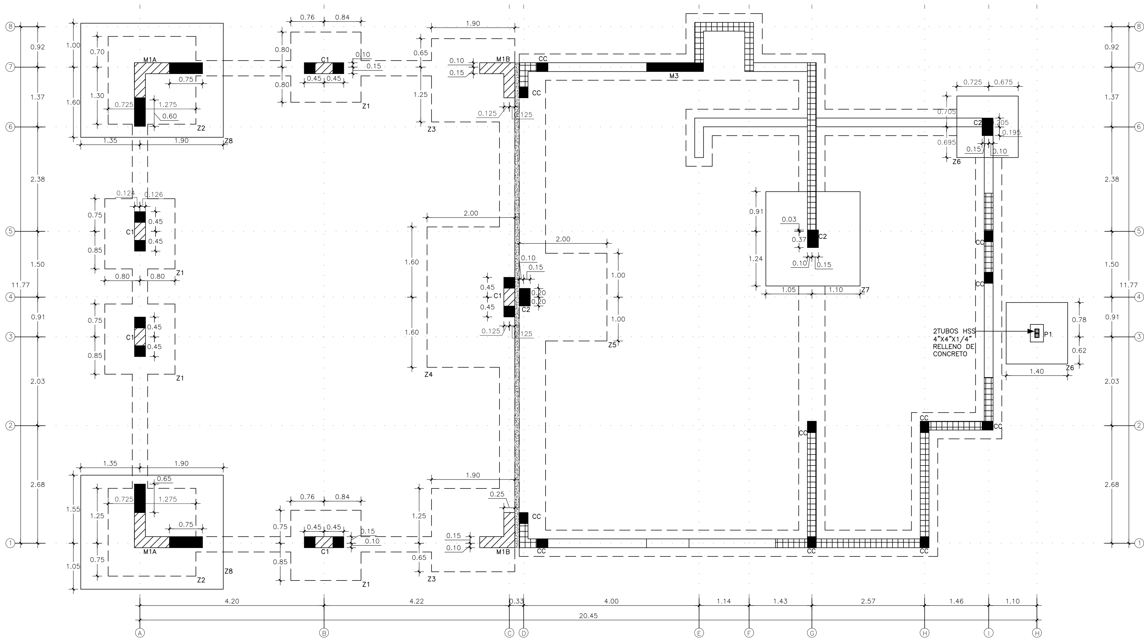
2 PLANTA ESTRUCTURAL DE REPLANTEO ESC. 1:50
