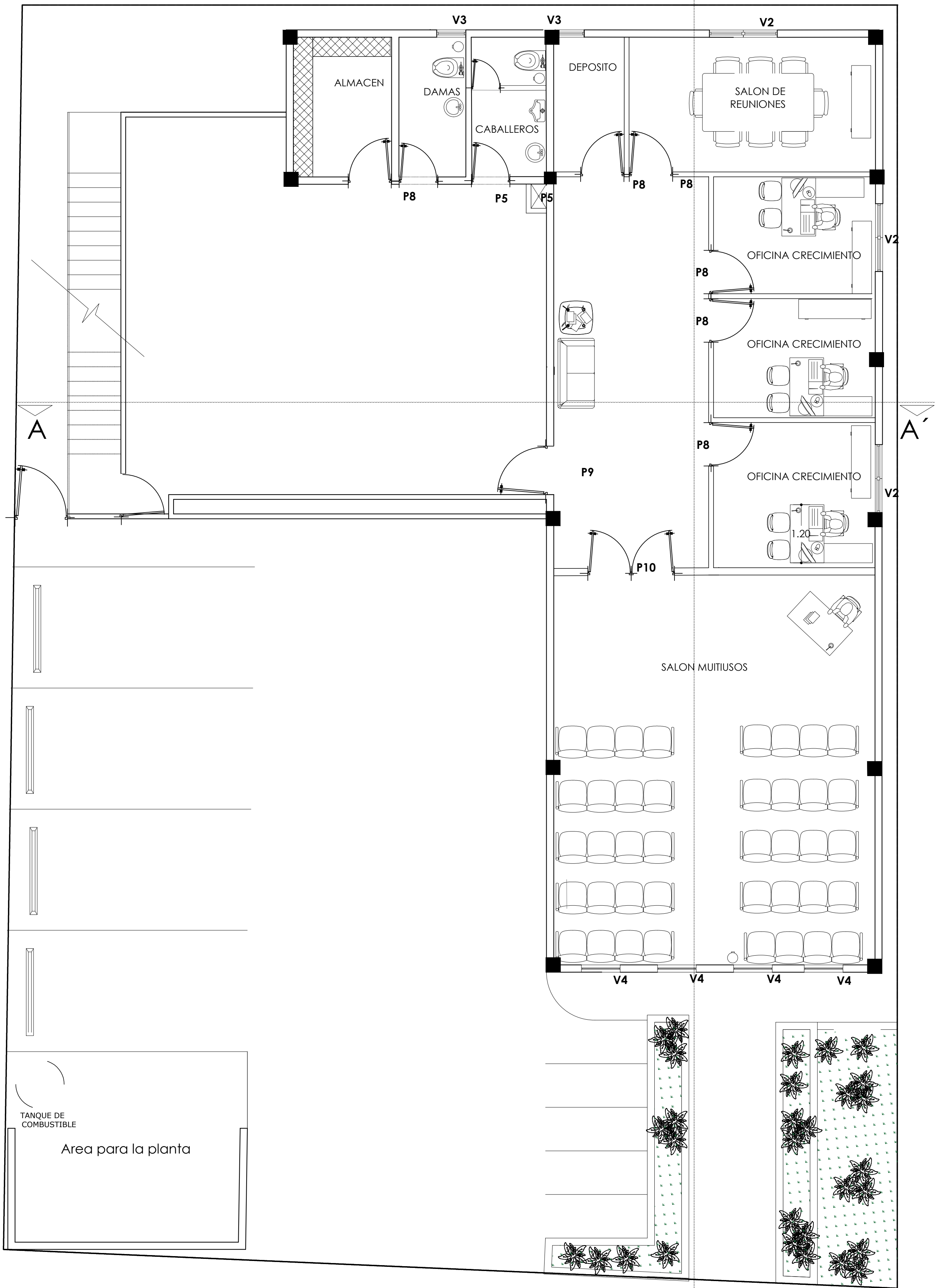
PLANTA DE PUERTAS Y VENTANAS 2DO NIVEL Escala: Indicada
